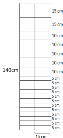
Stålstängsel 140cm/20/15
