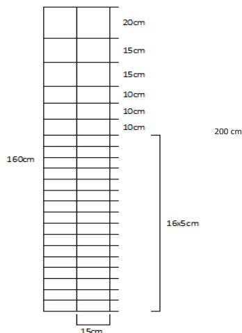
Stålstängsel 160cm/23/15
