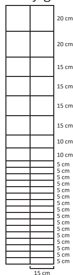
Stålstängsel 200cm/25/15
