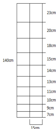
Stålstängsel 140cm/11/15
