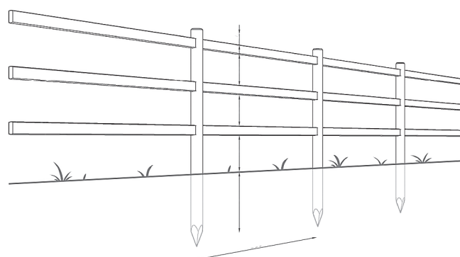
Colorado-hegn med 3 lægter
