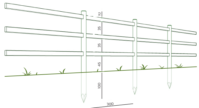
ColoradoZaun mit 3 Riegeln Verschiedene Zaunhöhen möglich
