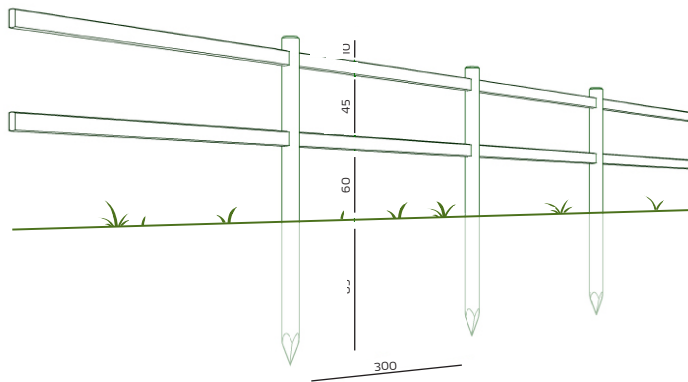
ColoradoZaun mit 2 Riegeln Verschiedene Zaunhöhen möglich
